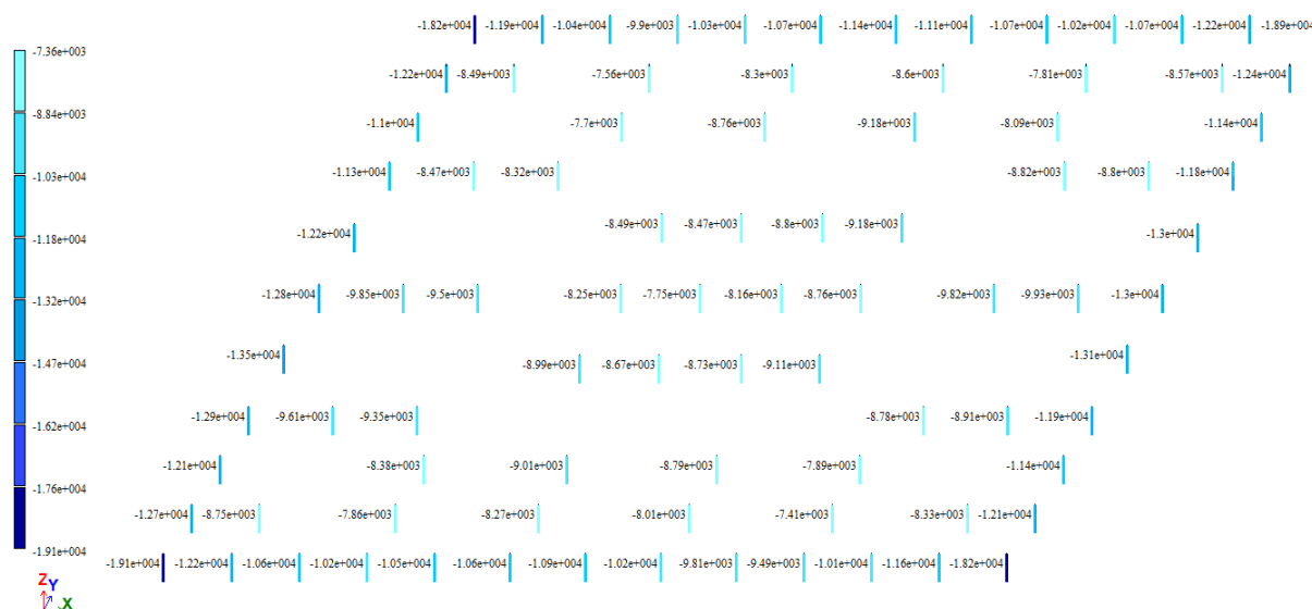
Рисунок. Усилия в сваях при учете работы основания.
