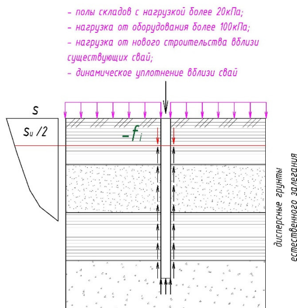
Случай висячей сваи с отрицательным трением
