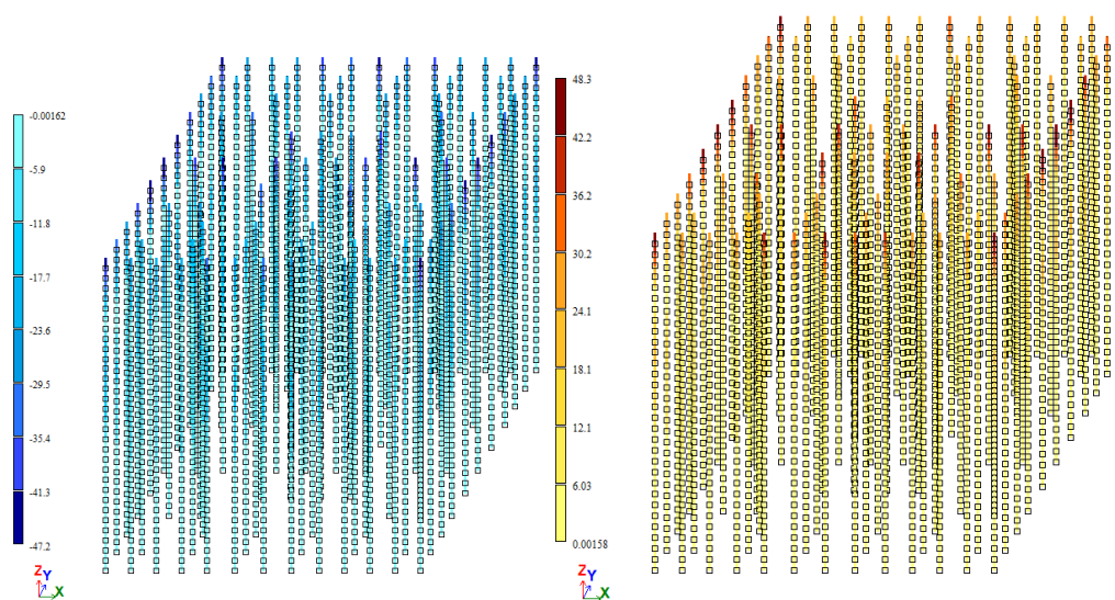
Минимальные и максимальные значения Q_y по РСЧ в сваях(кН)
