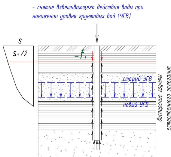
Случай висячей сваи с отрицательным трением
