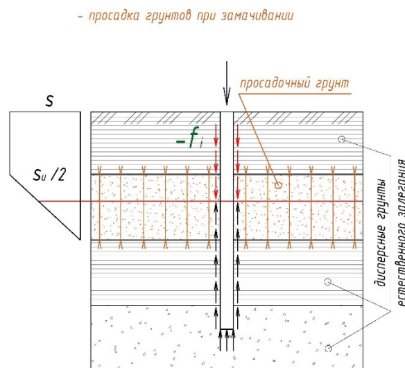
Случай висячей сваи с отрицательным трением
